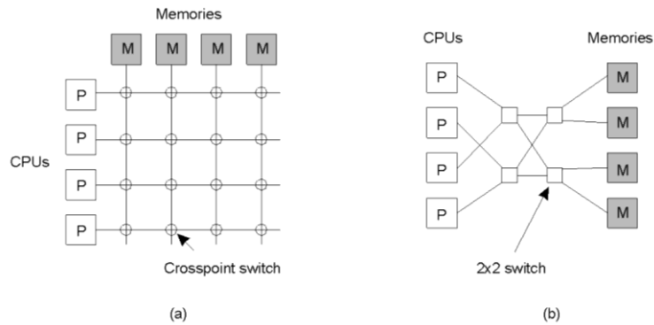
a) Křížový přepínač b) Omega přepínaná síť
