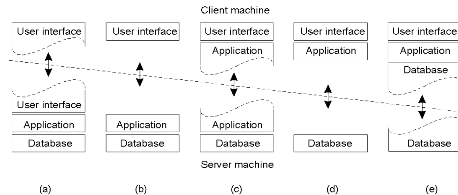
Alternativní organizace klient-server (a) – (e).
